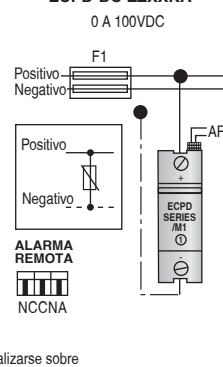
DIAGRAMA DE CONEXIÓN ECPD-DC-ZZXXKA
