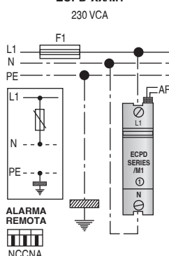
DIAGRAMA DE CONEXIÓN ECPD-XX/M1
