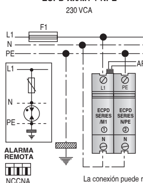
DIAGRAMA DE CONEXIÓN ECPD-XX/M1 + NPE
